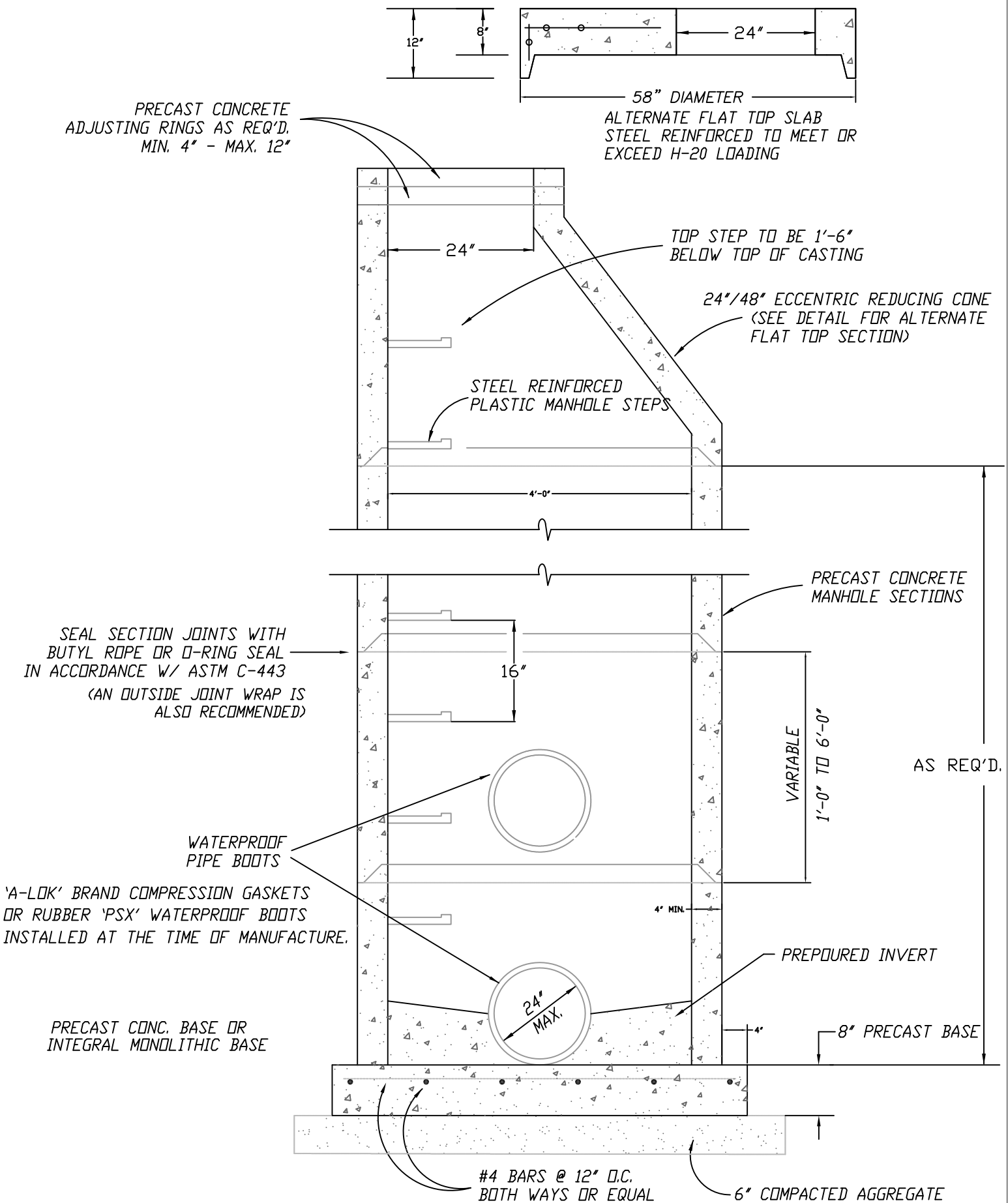
TYPE C MANHOLE
